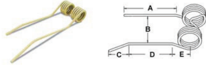
A-PZ224 Tedder Tooth
