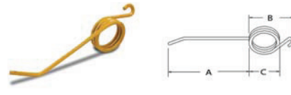
A-241379R Baler Tooth, RH
