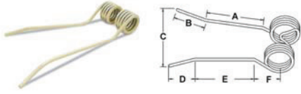
A-PZ225 Tedder Tooth
