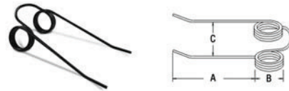
A-142856 Rake Tooth
